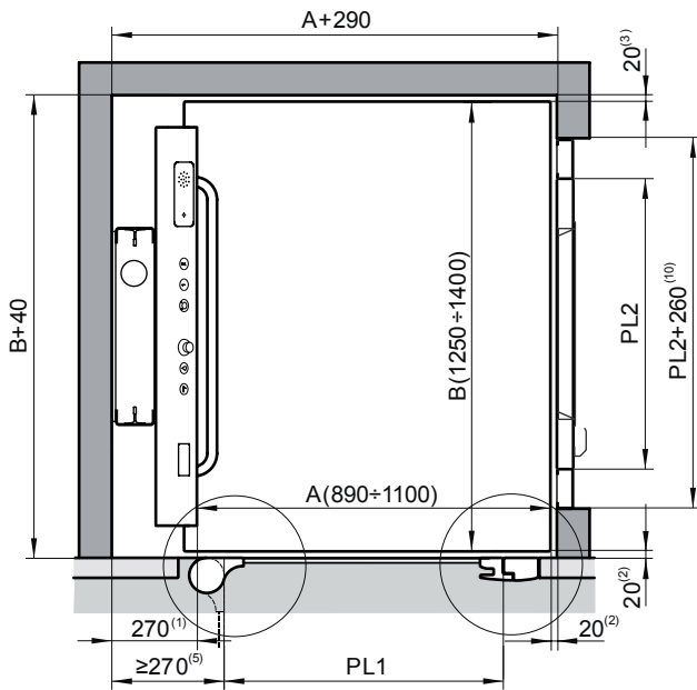
Doble embarque a 90° con acceso inferior frontal y puerta batiente sin dintel en nivel superior
