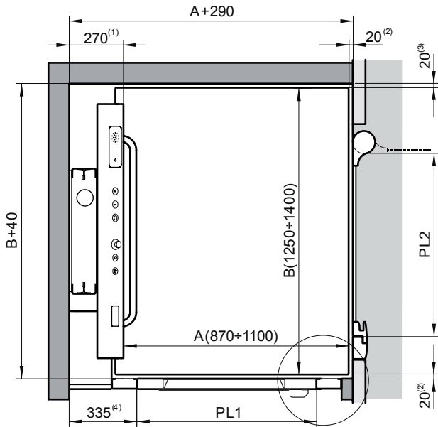
Doble embarque a 90° con acceso inferior lateral y puerta batiente sin dintel en nivel superior
