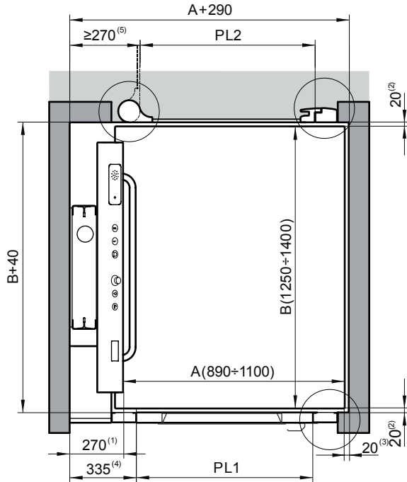
Doble embarque a 180° con puerta batiente sin dintel en nivel superior
