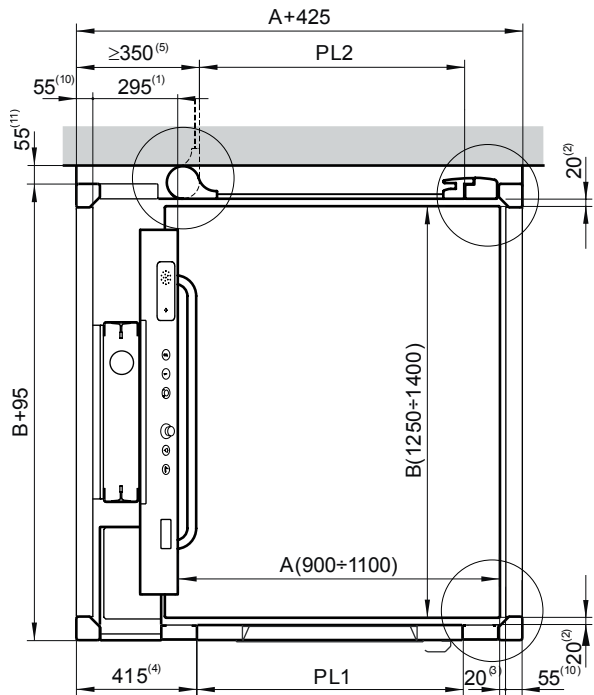
Cerramiento de cuatro laterales con puerta de altura 1100 en el nivel superior
