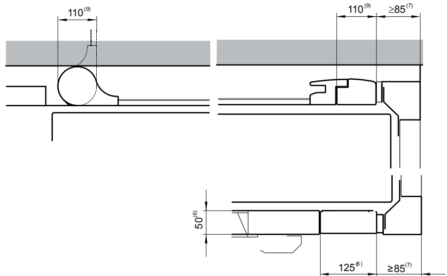
Cerramiento de cuatro laterales con puerta de altura 1100 en el nivel superior
