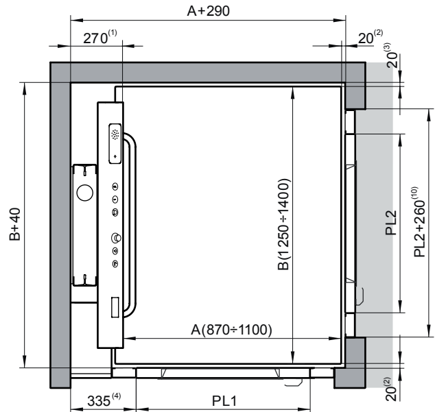
Doble embarque a 90° con acceso inferior lateral y puerta batiente de altura 2000 en nivel superior
