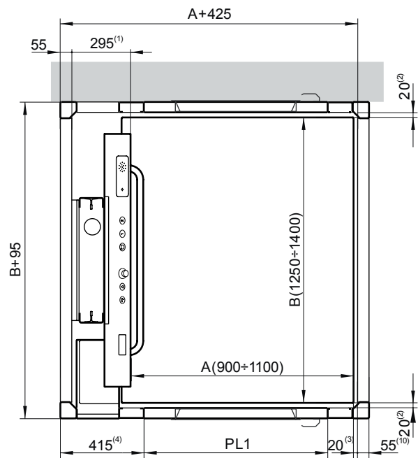
Cerramiento de cuatro laterales con puerta batiente de altura libre en el nivel superior
